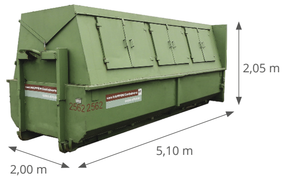
Haakcontainer gesloten 15 m 3
