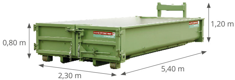
Haakcontainer open 11 m 3
