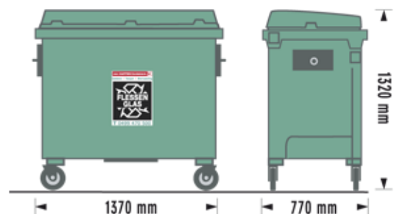
Rolcontainers staal 1300 Liter
