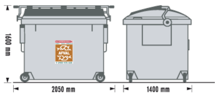
Gaascontainers metaal 1700 Liter
