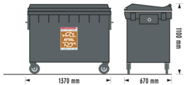
Rolcontainers kunststof 770 Liter
