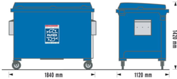
Rolcontainers staal 5000 Liter
