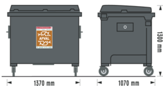
Rolcontainers kunststof 1100 Liter
