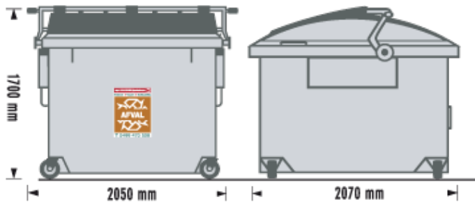
Gaascontainers metaal 2500 Liter
